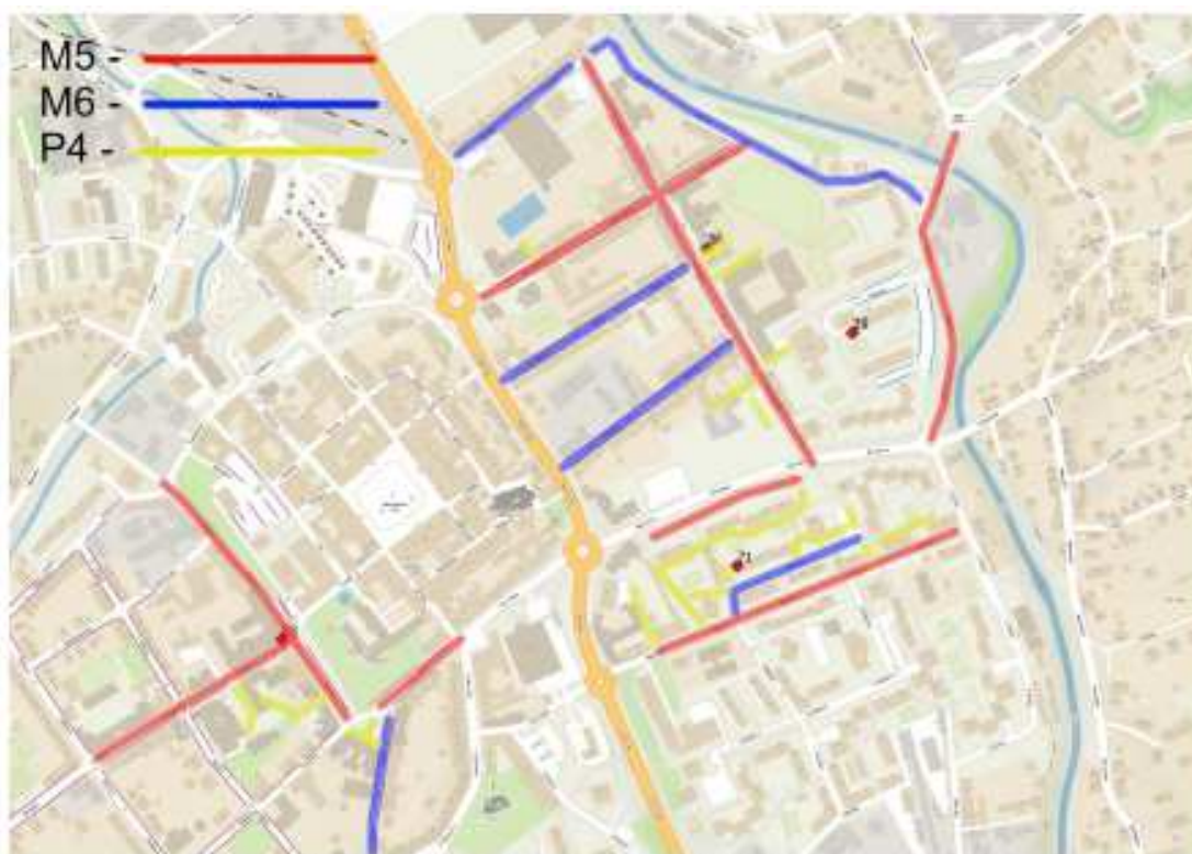
Zatřídění komunikací dle ČSN CEN/TR 13201-1 „centrum“
